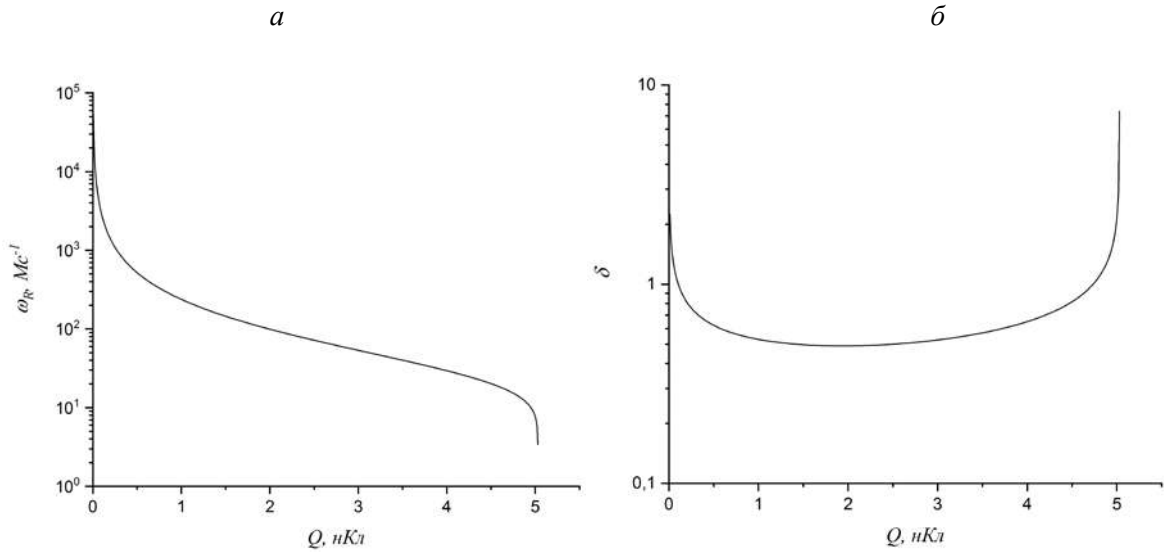
Рис. 4. Зависимости собственной частоты колебаний (а) и декремента затухания (б) для устойчивых радиусов от заряда на пузырьках при p_0 = 0.1 МПа, p_{v0} = 0.219 МПа, T_0 = 396.12 К.
