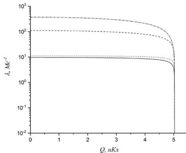
Рис. 3. Зависимость инкрементов неустойчивых равновесных радиусов от заряда пузырька при p_0 = 0.1 МПа, p_{v0} = 0.219 МПа, T_0 = 396.12 К: сплошная линия — общее решение уравнения (2.9), точечная, штриховая и штрихпунктирная линии — решения уравнения (2.9)
