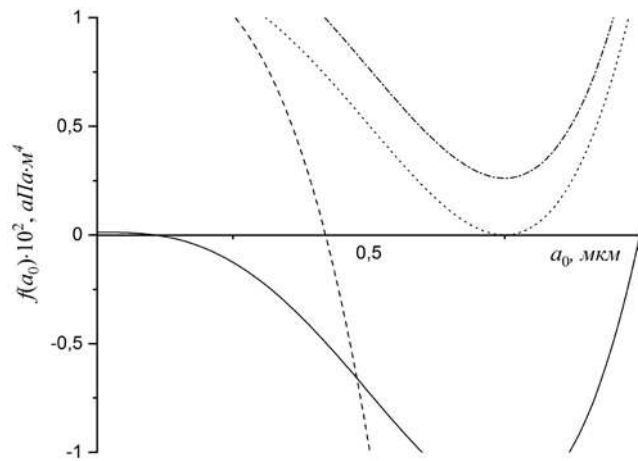
Рис. 1. Равновесные радиусы в зависимости от заряда паровых пузырьков: 1 случай - штриховая, 2 случай - штрихпунктирная кривая, 3 случай - точечная, 4 случай - сплошная.
