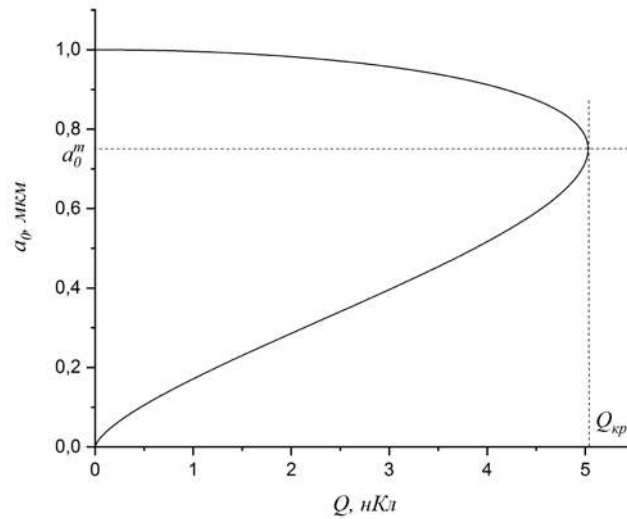
Рис. 2. Зависимость равновесного радиуса от заряда парового пузырька в перегретой воде при p_0 = 0.1 МПа, p_{v0} = 0.219 МПа, T_0 = 396.12 К.
